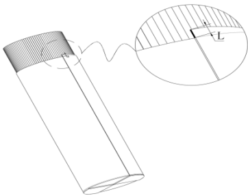
图1 包装纸对齐度测量示意图
